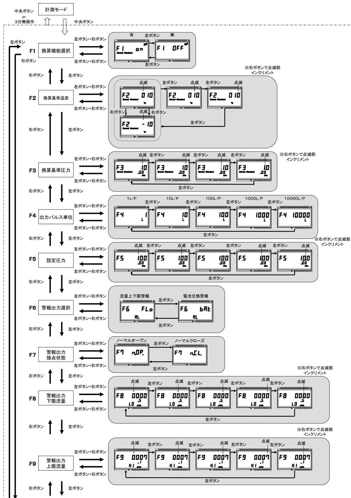
図 8 - 5. 各種設定モードの表示切替図(内蔵電池仕様)
