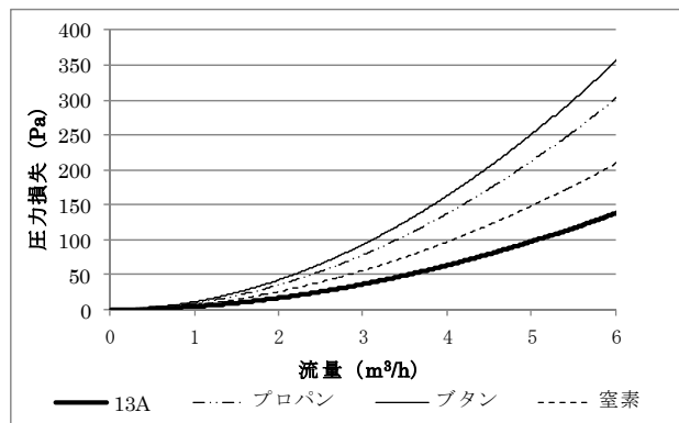
グラフ. 圧力損失 25A
