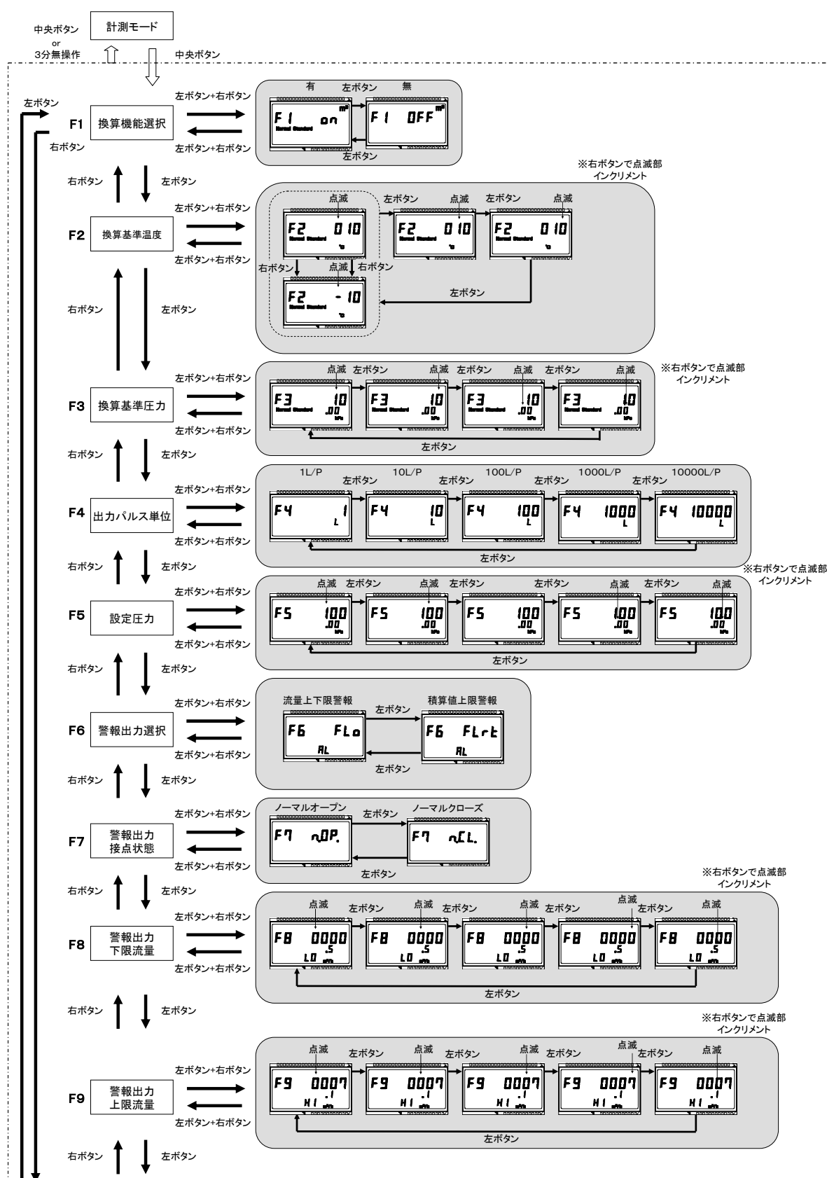
図 8 - 3. 各種設定モードの表示切替図(外部電源仕様)
