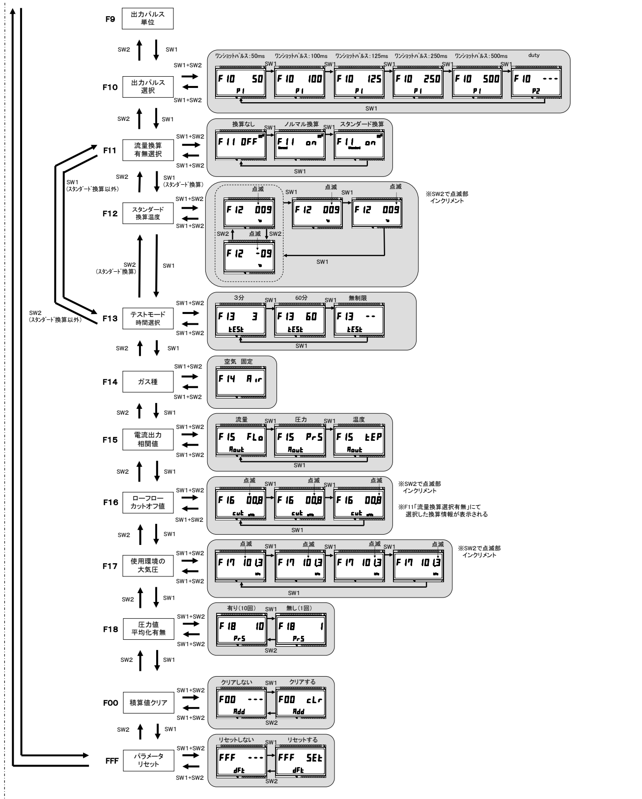
図 2-2 設定モードの表示切替フロー (B、D) (2/2)
