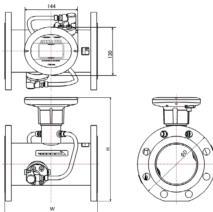
图 10-1 外形图
