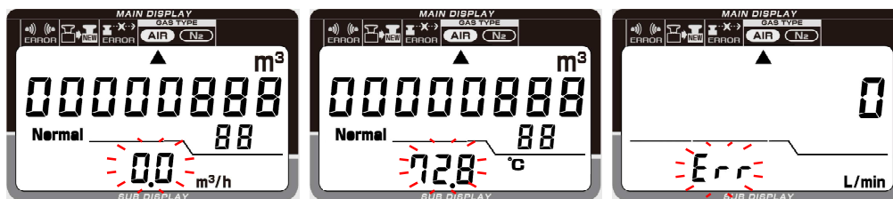
図 6-3 温度異常表示
